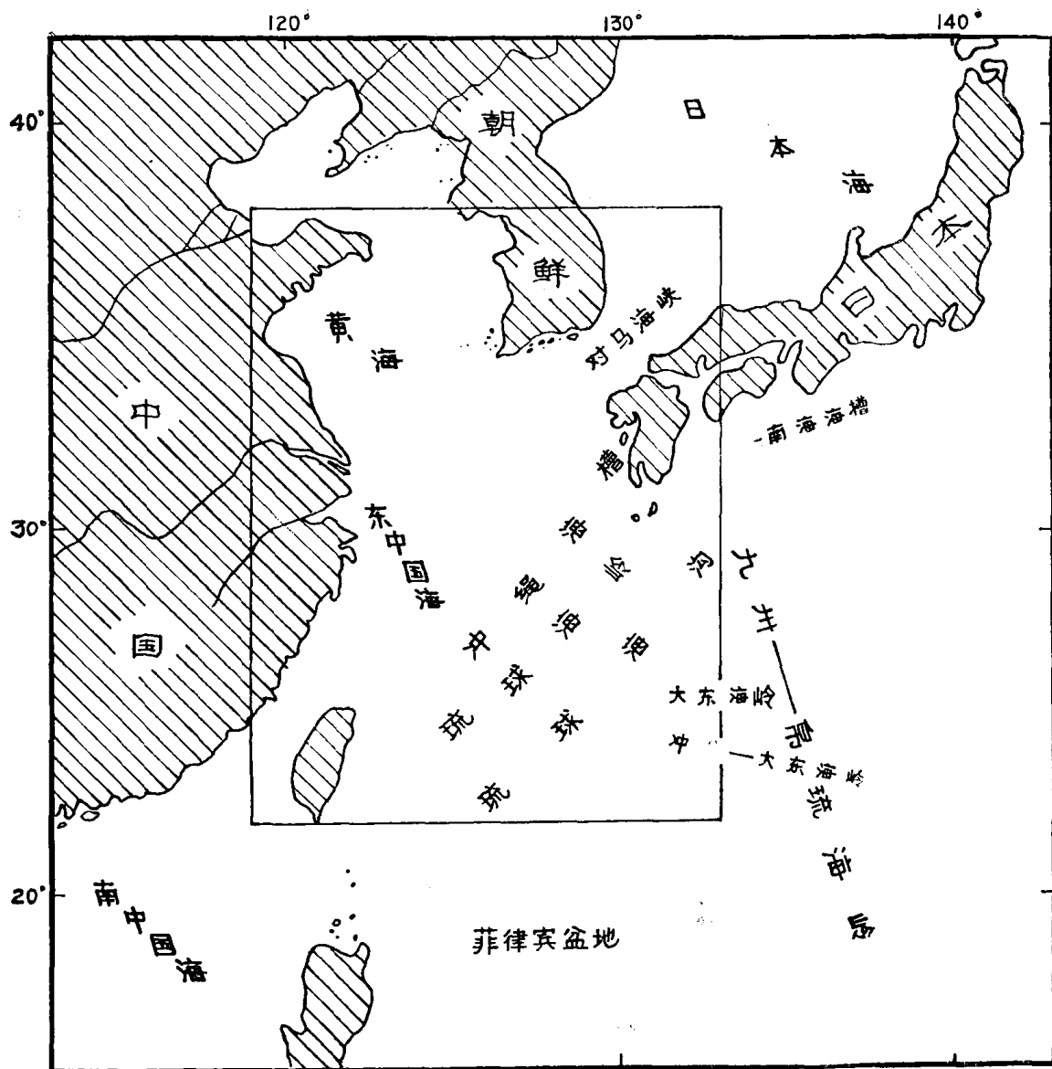
图 1 东亚地球物理调查位置图
