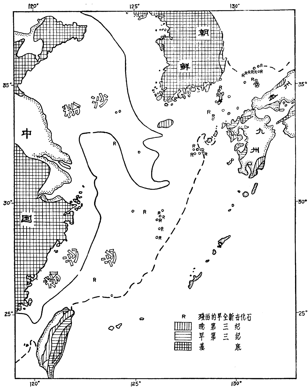
图 3 东中国海和黄海海底底质分布略图
