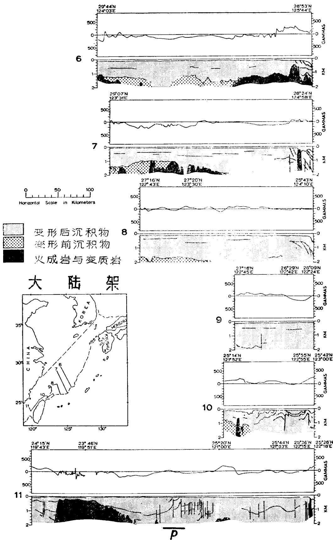
图 9 东中国海大陆架西南部的连续地震反射剖面 and 地磁剖面解释
