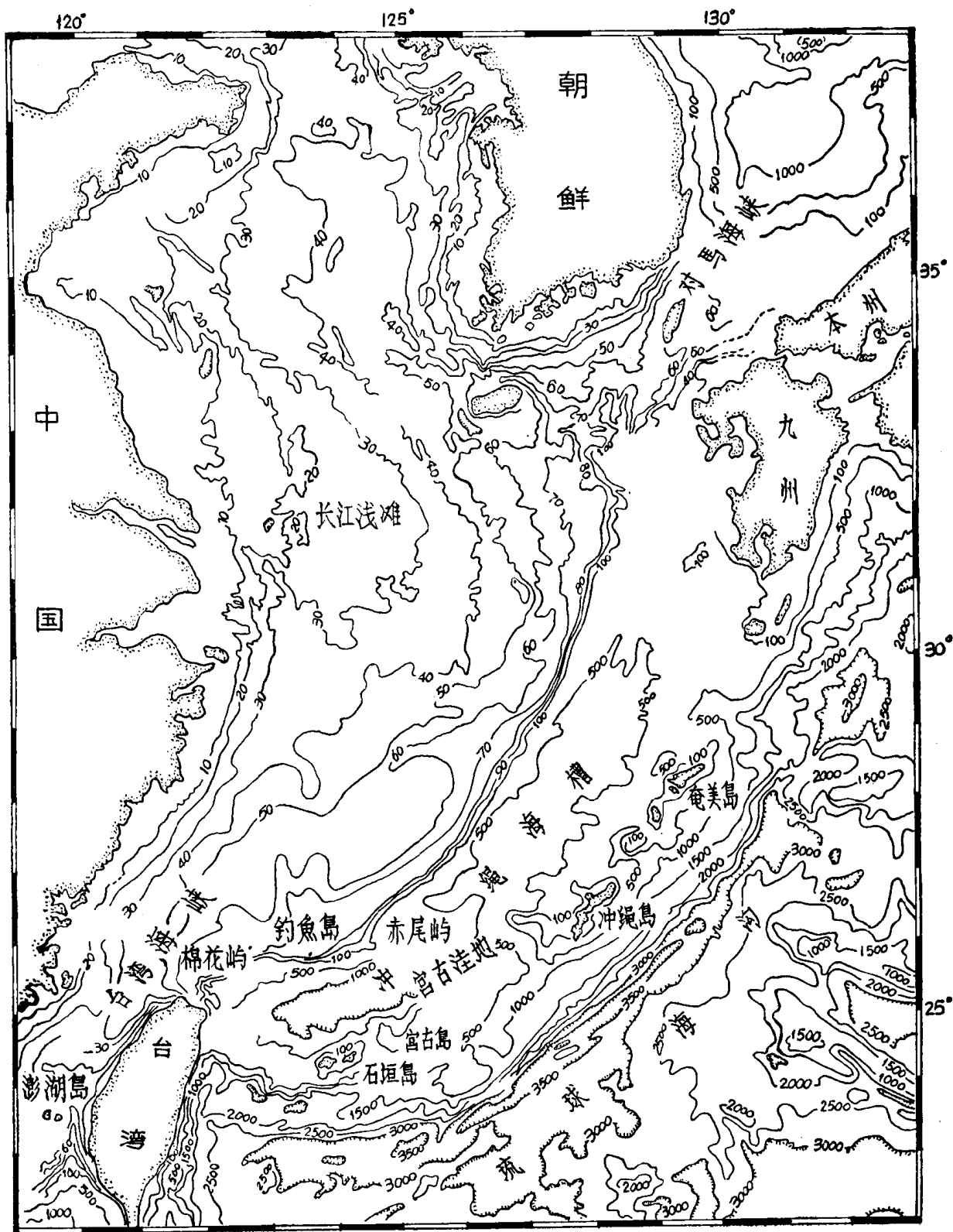
图 2 东中国海和黄海海底地形图
