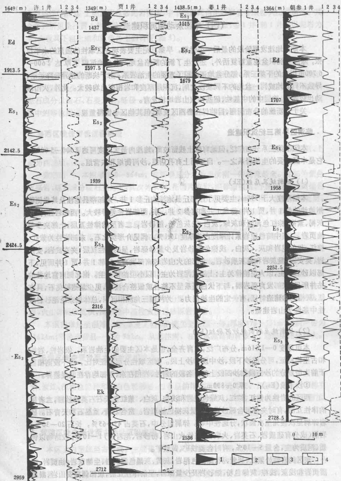
图4 莘县地洼下第三系沉积韵律、碎屑粒度、泥岩颜色参数曲线图 (图例同图2)
