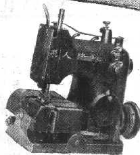
146-1型縫袋用縫紉機 供製棉織化工織品及織物等用
