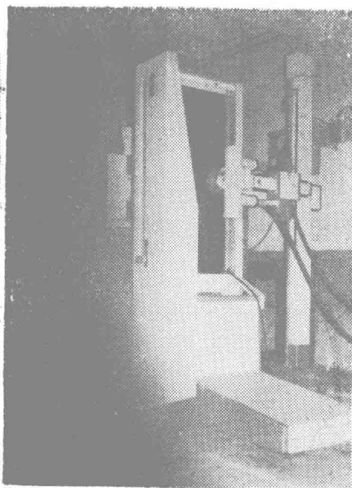
瓦寨区卫生院100毫安射线机
