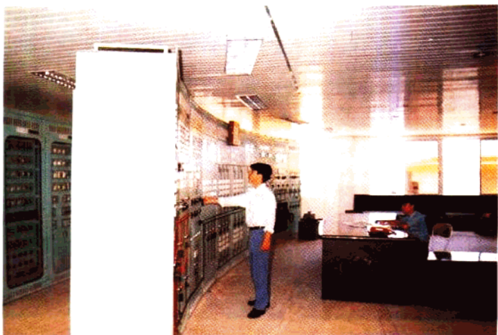
▲海安开发区 110 千伏变电站中控室
