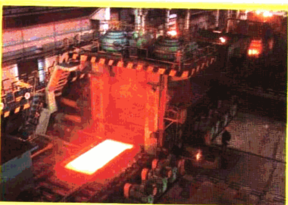
1989 年 1 月建成并投产的中板四辊轧机生产线
