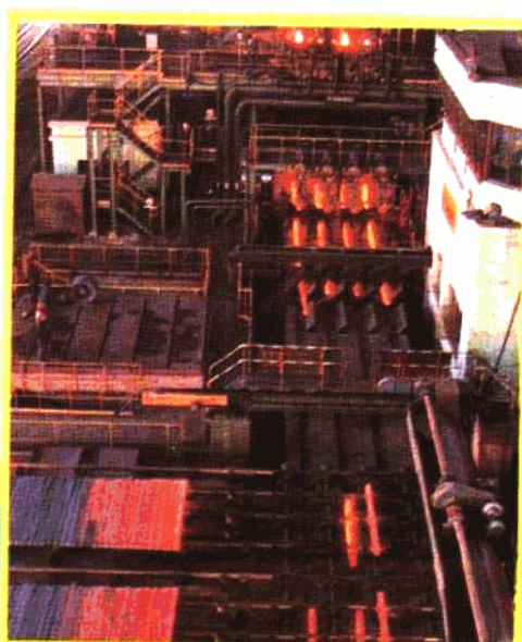
1988 年从意大利引进的四流方坯连铸机生产线
