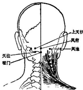
图 1-5 项部穴位
