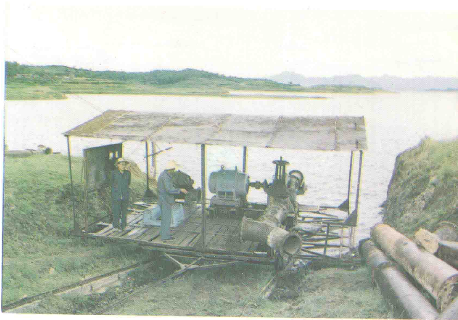
能升能降的黑卧扬水站
