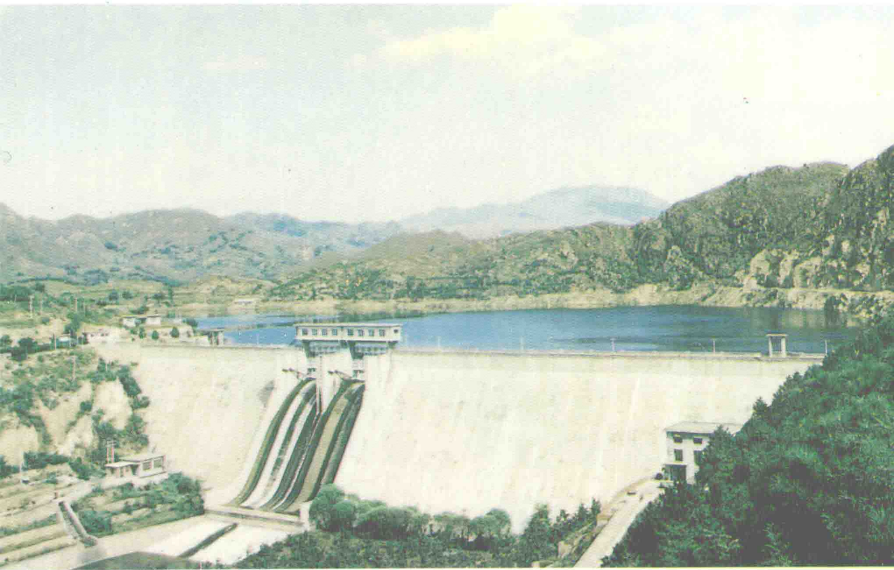
密云县第一座中型水库——沙厂水库
