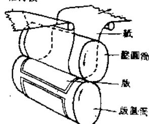
圖 1.1.2 印刷機的三種形式 (取材於馬漢務之印刷入門)
