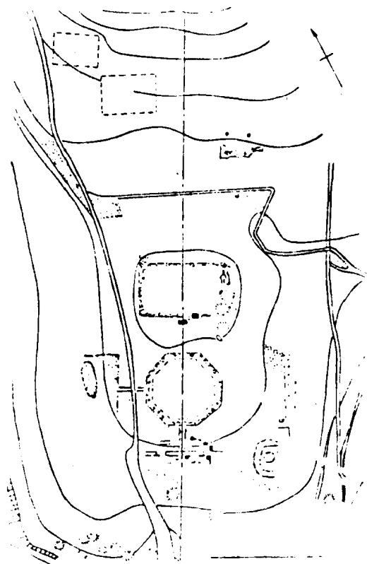
图一三 金刚寺遗址平面图
