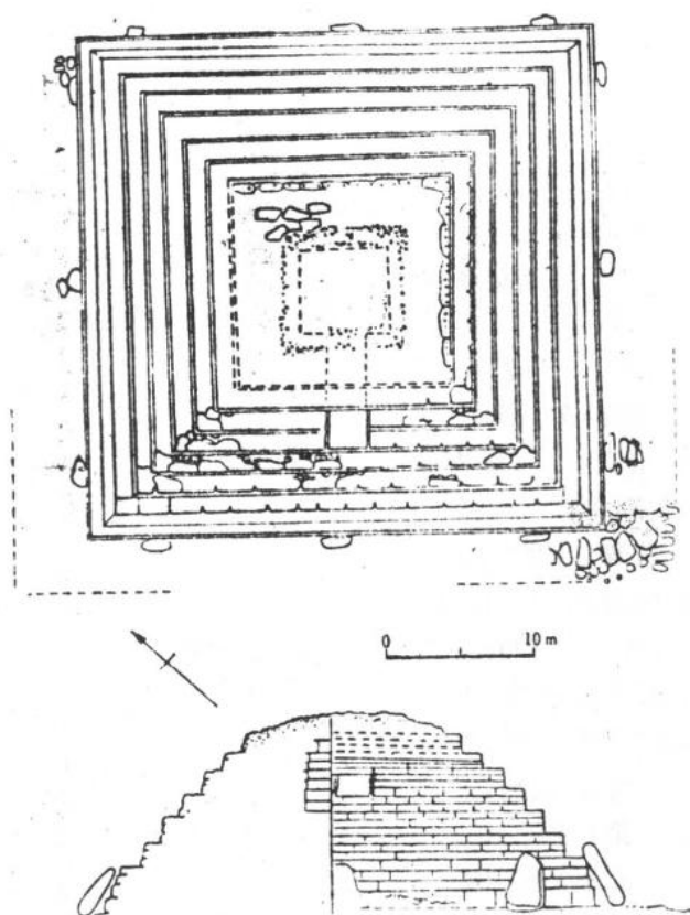
图一〇 将军坟平面、断面图
