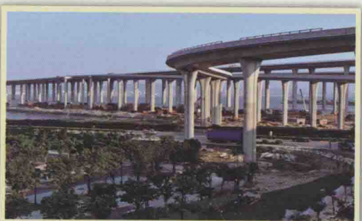
杏林公铁大桥 于2006年3月动工建设，2008年9月1日建成通车，公路、铁路两用通道。大桥全长8.53公里，主桥设计为驼峰桥。
