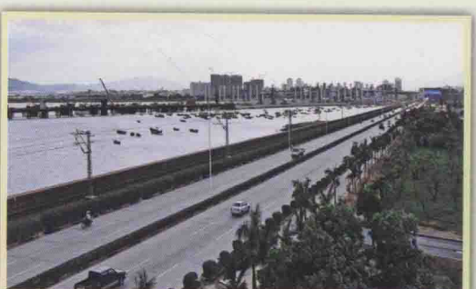
集杏海堤 于1956年底建成，全长2820米。当时修建的鹰厦铁路将海岛厦门与大陆连接起来，作为当年修建鹰厦铁路的“咽喉”工程。
