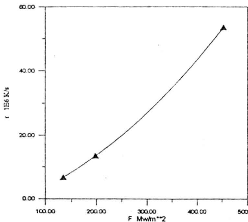
图 3 金属薄膜中心点处的温升速率 r 与 F 的关系曲线
