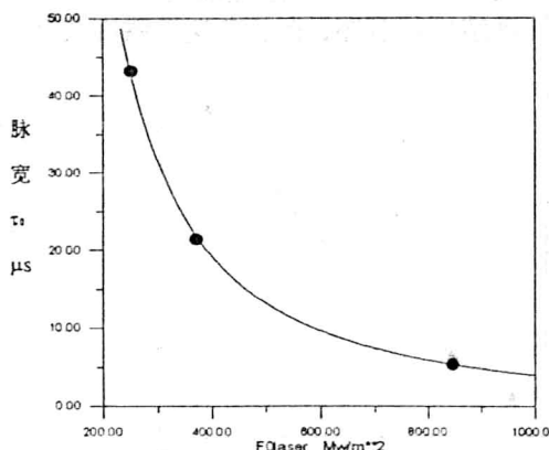
图 10-2 与激光能量密度 F_{laser} 对应的脉宽 \tau
