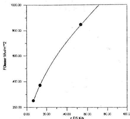
图 10-1 温升速率 r 与人射激光能量密度 F_{laser} 的关系
