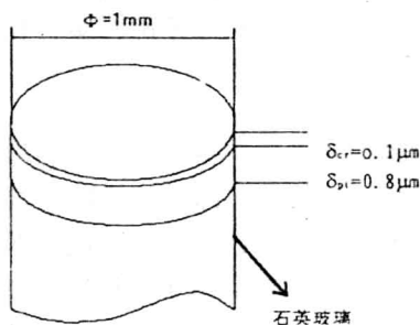
图 1 实验件结构示意图
