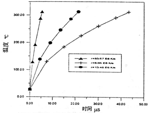
图 7 不同温升速率下表面温度的变化过程
