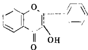
黃醌醇 (flavonol)
