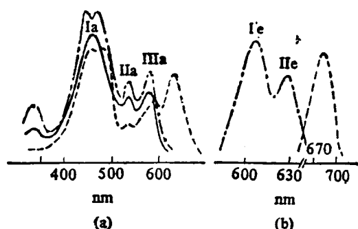
图1 HA 的吸收、激发和荧光光谱
