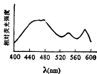
图 4 HA 的荧光激发光谱
