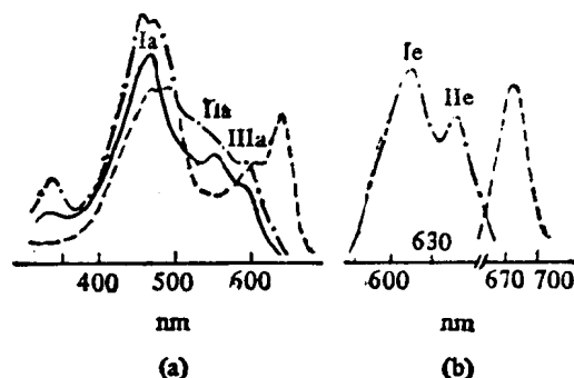
图2 HB 的吸收、激发和荧光光谱
