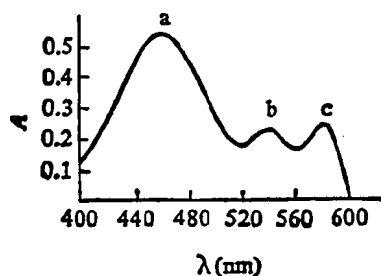
图 3 HA 在无水乙醇中的吸收光谱
