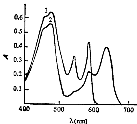
图 5 HA 的可见吸收光谱 1. 77K; 2. 碱性溶液
