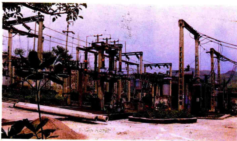
南川县城郊变电站一角。
