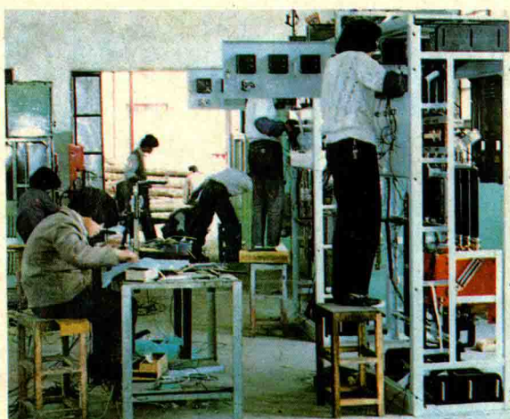
慈溪高压开关厂装配车间一角。
