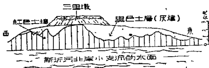
圖四：三里墩地層剖面圖
