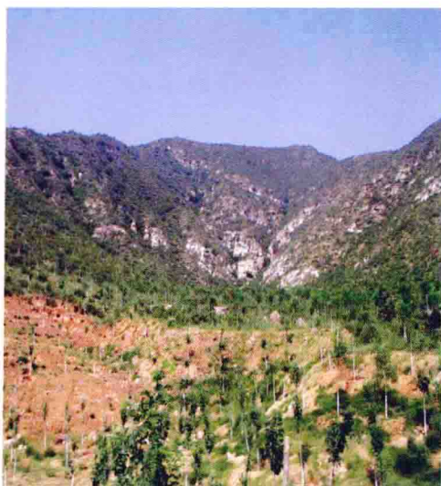
帮水峪西山爆破造林工程
