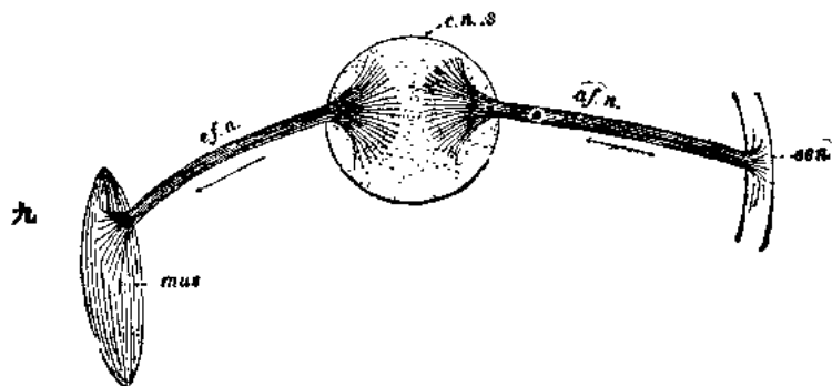
反 射 弧 之 圖
