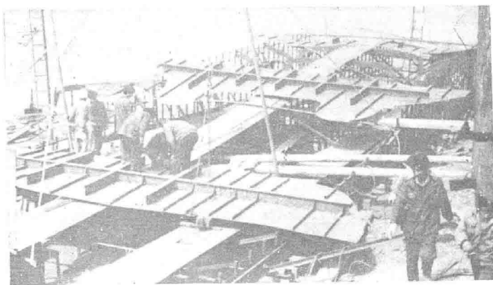
涪陵市城七校造船厂在万县建造60米中型豪华客轮 万州8号船底施工图。
