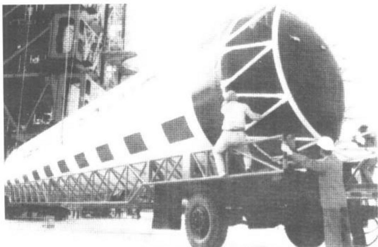
“长征四号”运载火箭。
