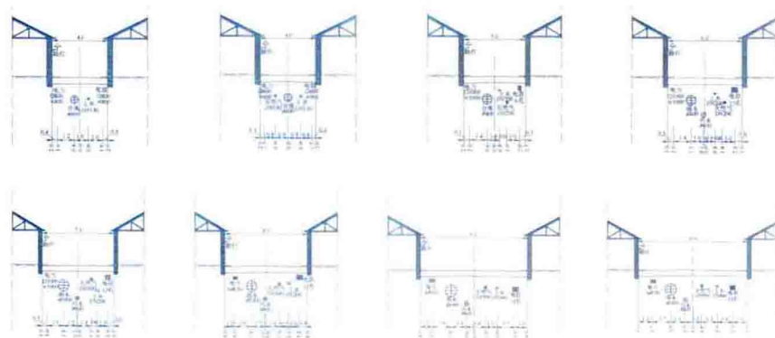
图13 不同宽度胡同市政管线断面设计示意图
