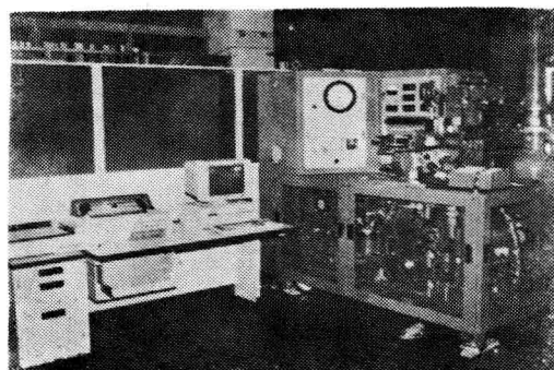
国内最先进的化油器综合流量试验台 (引进日本OVAL公司产品)
