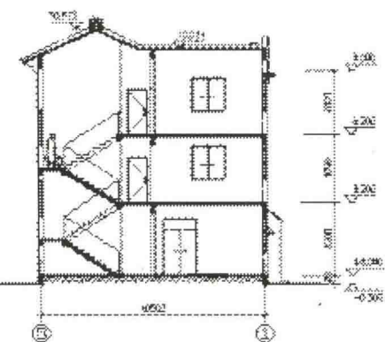
1-1 剖面图
