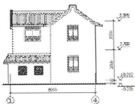
1-4 立面图
