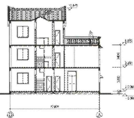
2-2 剖面图
