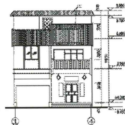
正立面图
