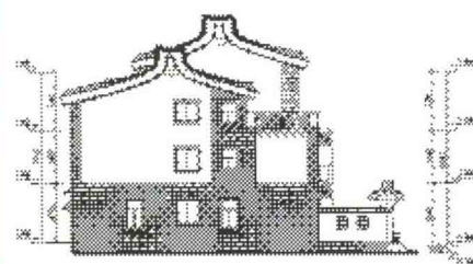
西立面图
