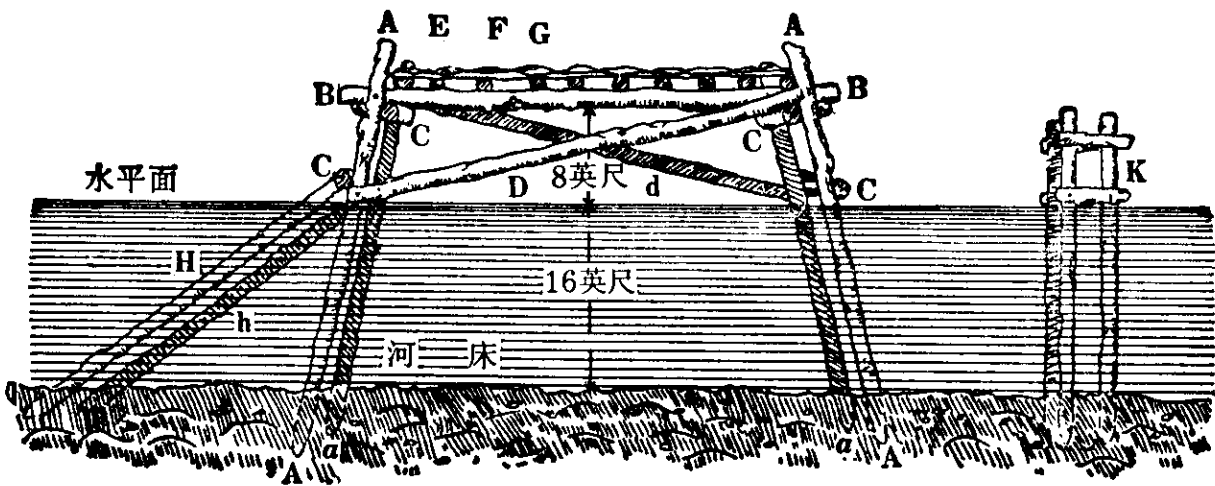
桥架截面图
