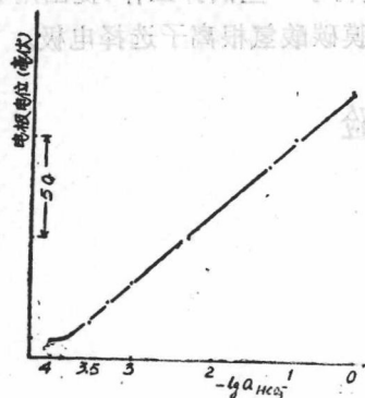
图1 电极响应曲线
