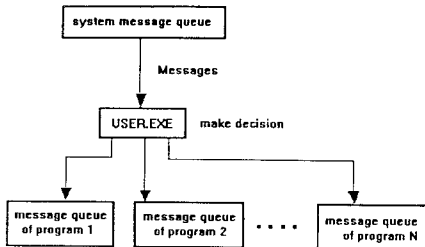
图 1.4 系统消息队列中的消息转移
