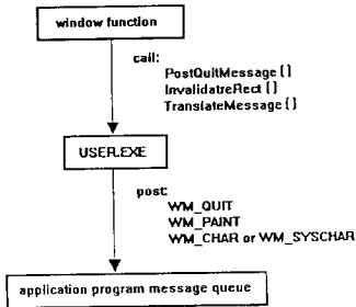
图 1.5 由 Windows 函数调用产生的消息
