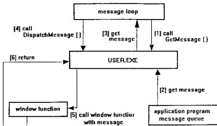
图 1.6 应用程序获取和处理消息的流程
