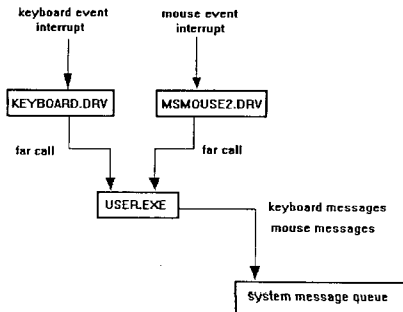
图 1.2 键盘或鼠标消息的产生
