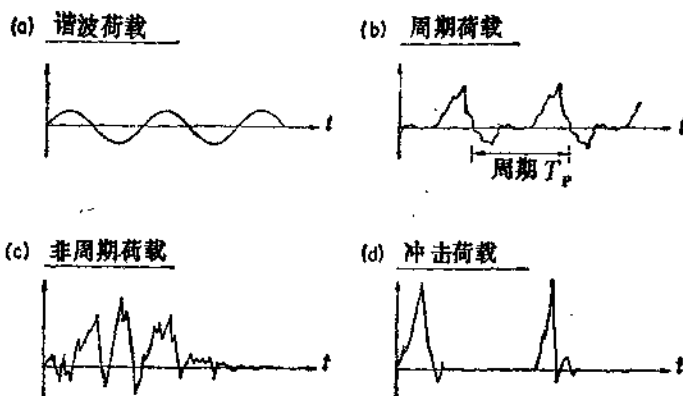
图 1.2 典型动荷载的时间函数
