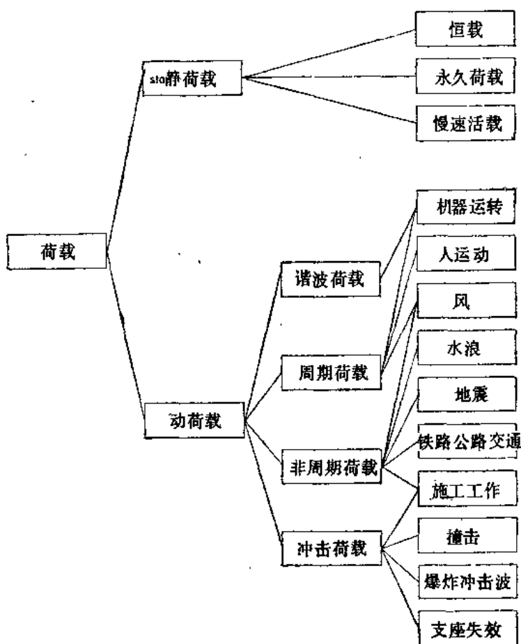
图 1.1 土木工程中的荷载类型
