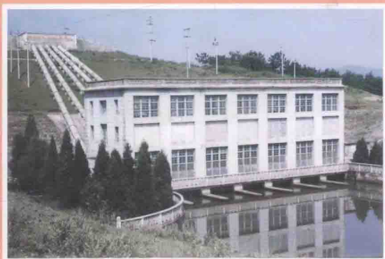
郑家湾一级泵站
