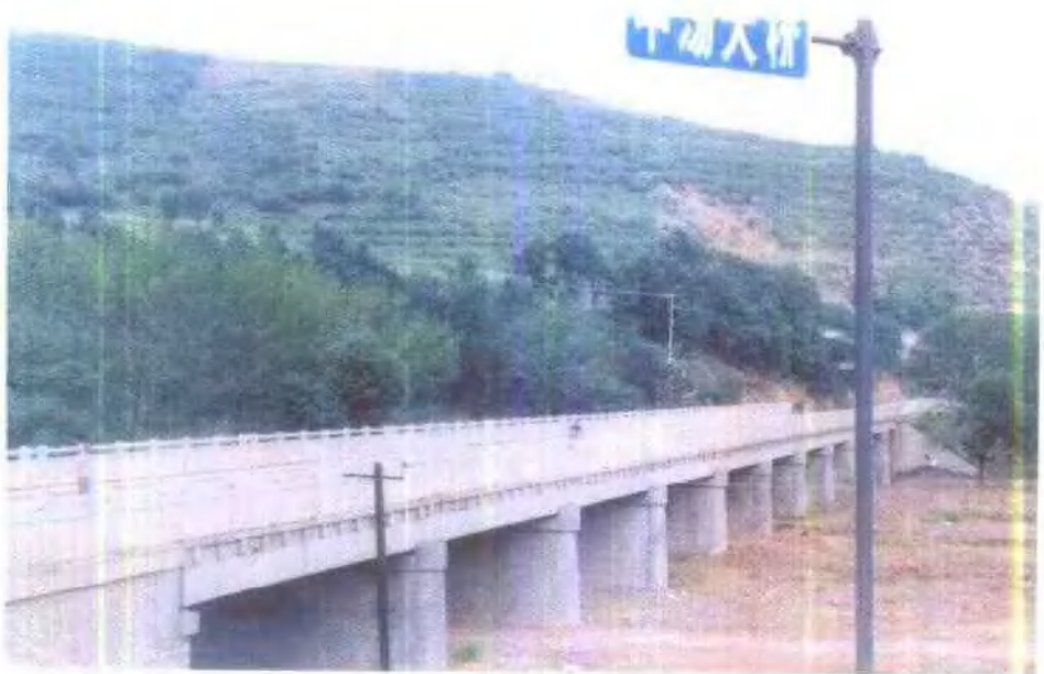
图为中汤大桥。该桥全长199.12米，宽9米，1995年11月15日开工，1996年10月1日竣工，总投资239万元。
