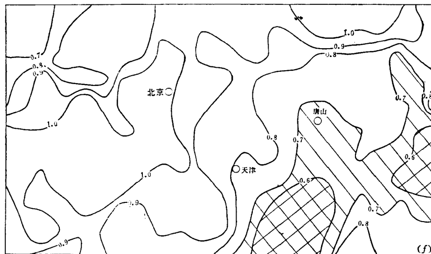
不同日期 b 值空间扫描
