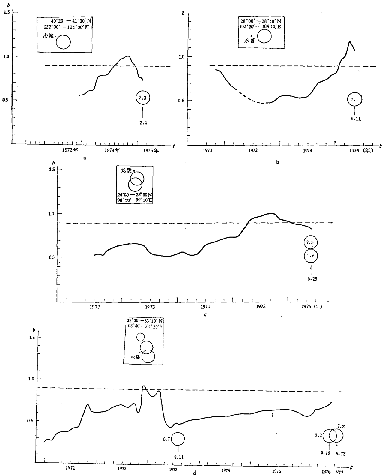
图 8 其它四次 7 级以上地震前 b 值时间扫描
