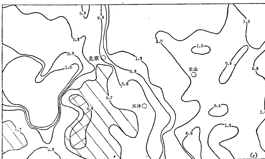
图5 京津唐渤海地区 (a) 1966.4.1—1968.3.31; (b) 1970.1.1—1972.12.31; (c) 1972.5.1—1974.4.30;
