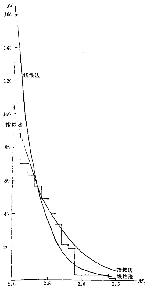
图 11 T_0 区 (1967 年 9 月 21 日—1969 年 9 月 12 日) 观测累计分布与指数及线性最小二乘拟合结果的比较
