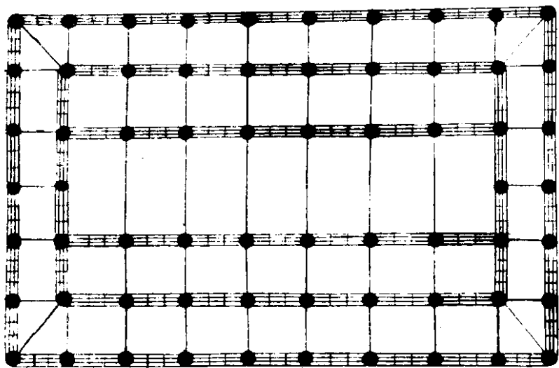
殿間地盤殿身七間副階 周市各兩架椽身內雙槽
