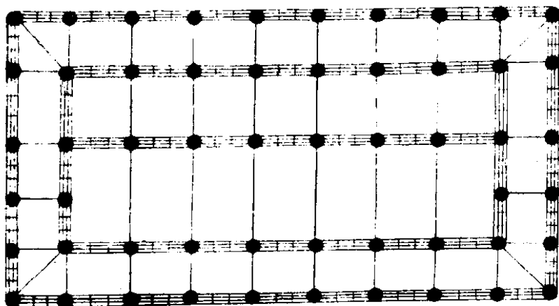
殿間地盤殿身七間副階 周市各兩架椽身內單槽
