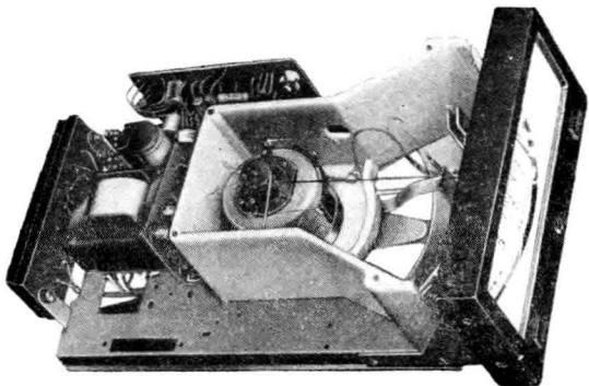
XCT系列 动圈式指 示调节仪 内观
