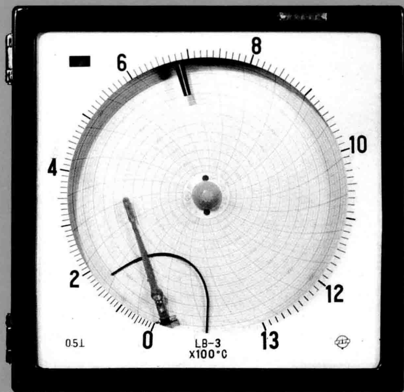
XWG系列中型圆图记录仪
