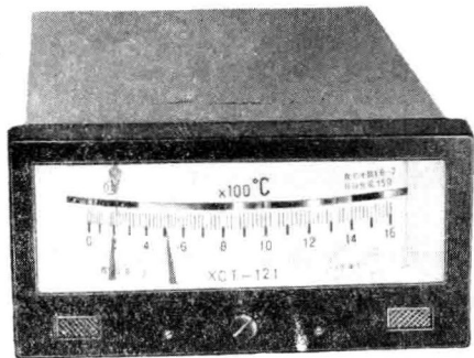
XCT系列动圈式指示调节仪外形
