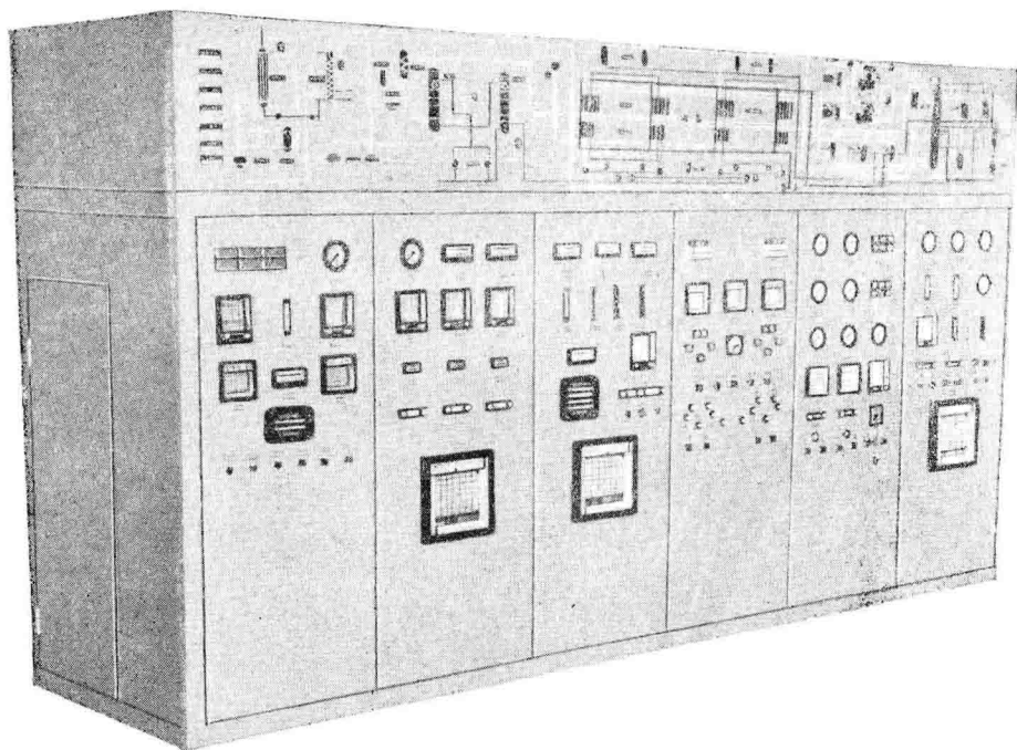
KG型柜式仪表盘(多盘并列，加模拟盘)
