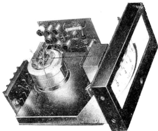
XCZ系列 动圈式指 示仪内观
