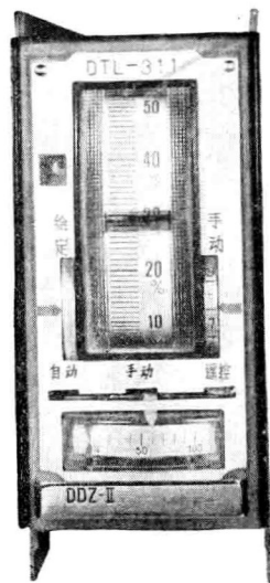
DTL-311型 比例积分微分调节器
