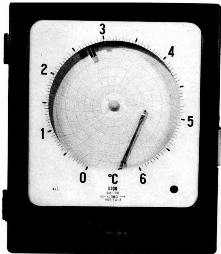
记录仪
