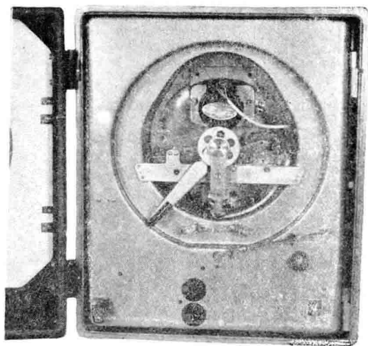
EWY-731型结晶定碳仪(表壳正面)
