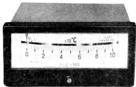
XCZ系列动圈式指示仪外形
