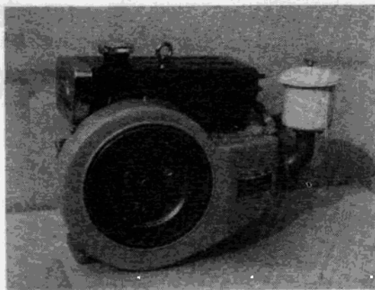
县柴油机总厂生产的 170L 天鹅牌柴油机
