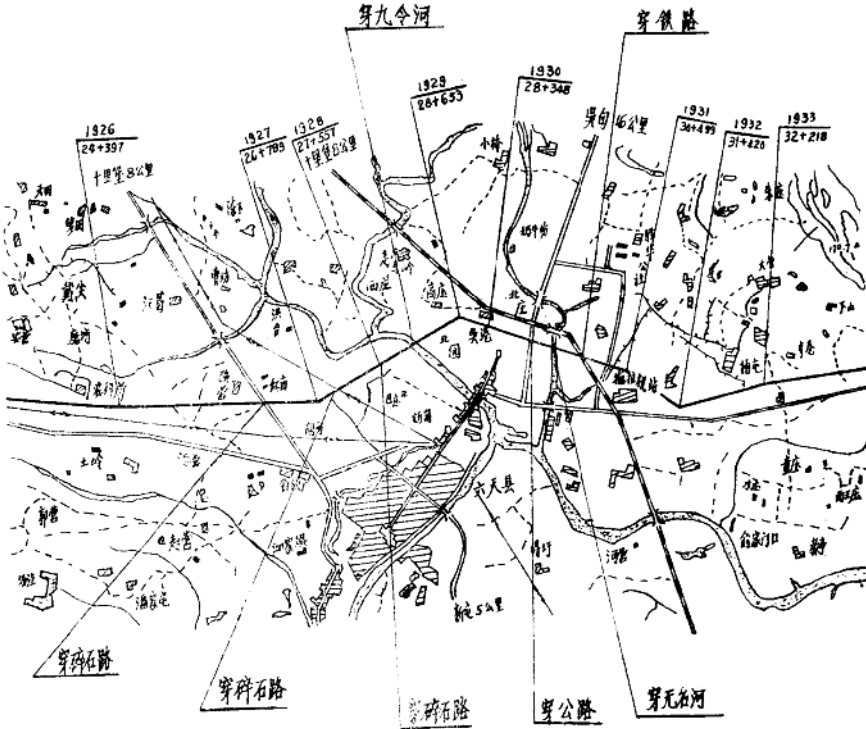
图1—2 输油管线平面图 (1 : 50,000)
