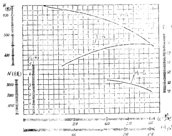
图2—1 DKS750—550型泵工作特性
