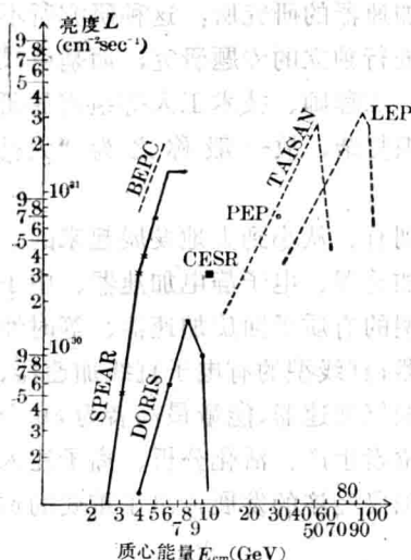
图1 储存环亮度与质心能量 E_{cm} 的关系
