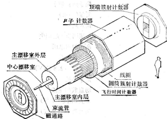
图 3 探测装置外形图
