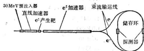
图 2 正负电子对撞机总体布置示意图
