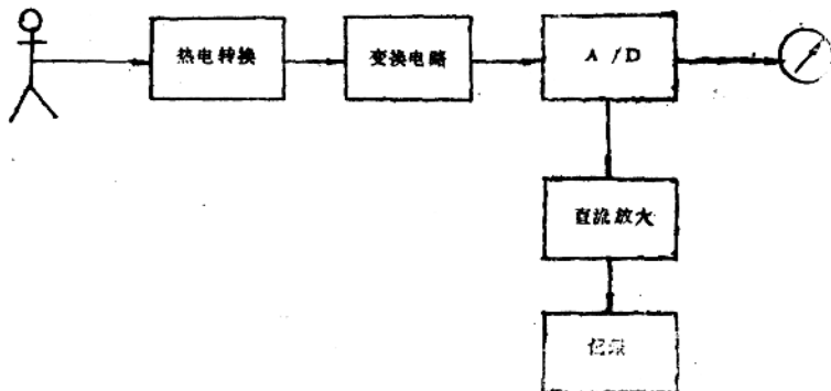
图 1-4 自动体温计
