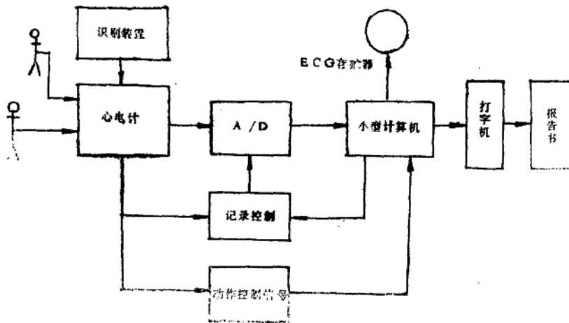
图1-6 心电自动解析装置图
