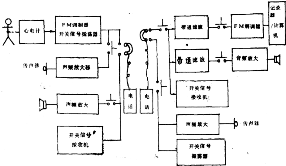
图 1-3 用电话线路传递心电图
