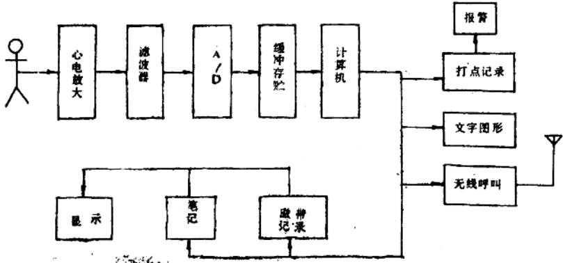
图1-7 全自动心电监护装置
