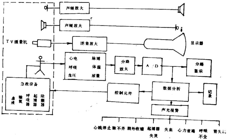
图1-8 全自动监护系统方框图
