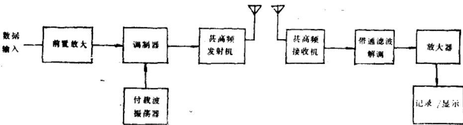
图1—2 医用数据无线传输
