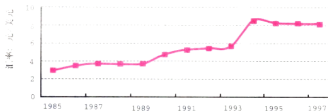
1986—1997年中国外债余额情况
