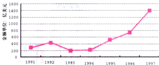
1991—1997年中国外汇储备情况
