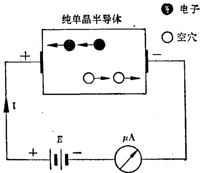
图 1-5 半导体中载流子的移动
