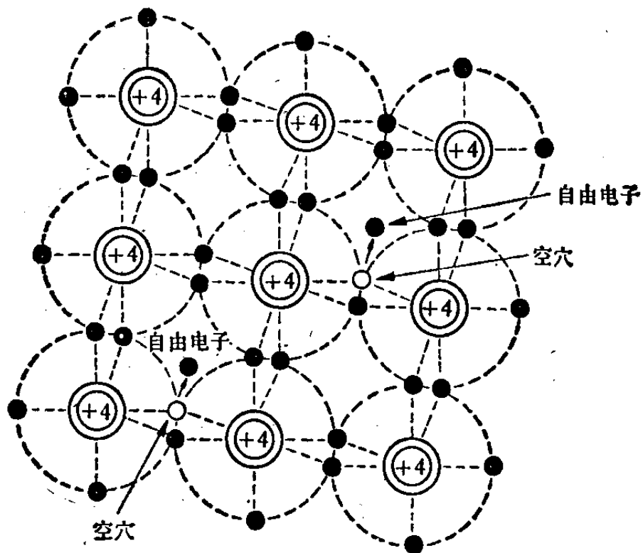
图 1-4 热运动产生的电子-空穴对
