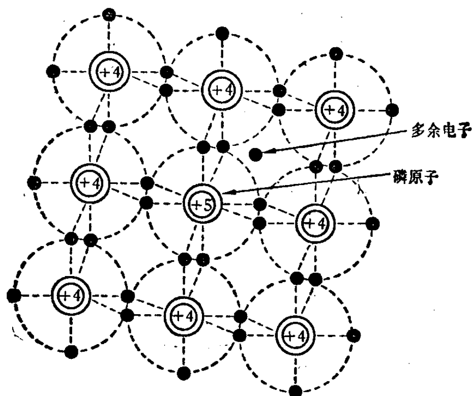
图 1-6 N 型半导体(硅掺入磷形成电子载流子)
