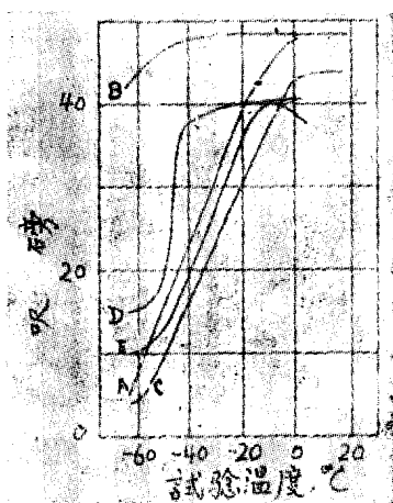
图 13 上表中钢的冲击转折温度曲线
