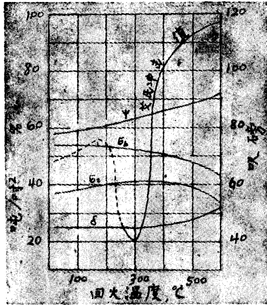
图9 回火温度对室温机械性能的典型曲线
