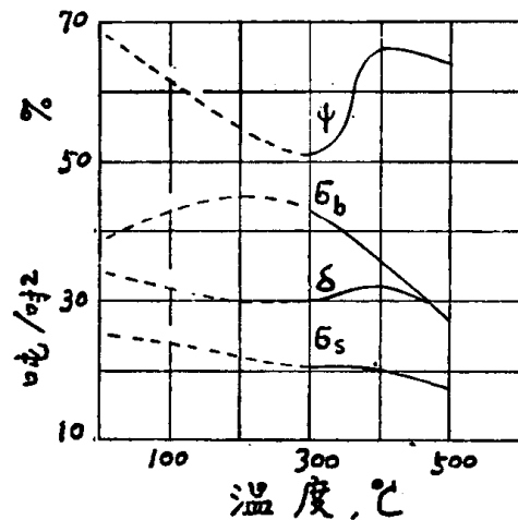
图 14 温度对 1 英寸直径钢 (%: 0.23C, 0.12Si, 1.67Mn) 棒 (810°C 正火) 机械性能的影响 [6]
