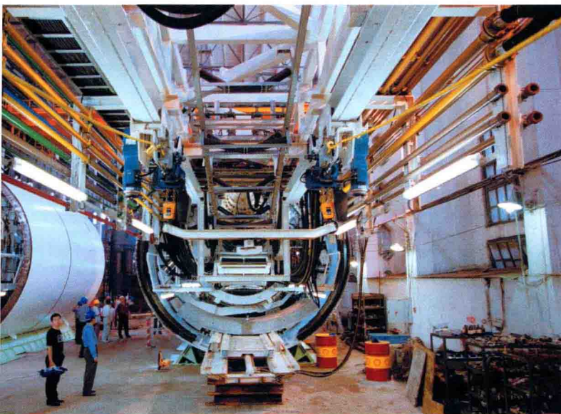
大型机械装备——盾构机生产车间
