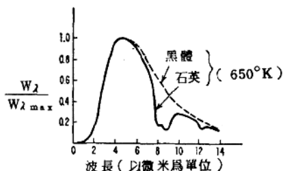
圖 1-4 650°C 時，石英晶體與黑體輻射能譜之比較
