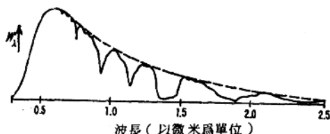
圖 2-3 太陽輻射能譜。(缺陷部分是由於大氣層的吸收所致)
