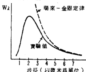
圖 1-1 黑體輻射曲線（實線所示為實驗所得結果，虛線部分是以古典理論導出的不正確的結果）
