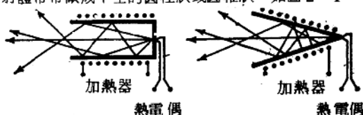
圖 2-1 圓柱狀和圓錐狀的空腔輻射體
