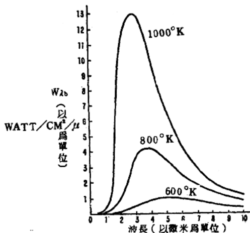
圖 1-3 黑體輻射能譜
