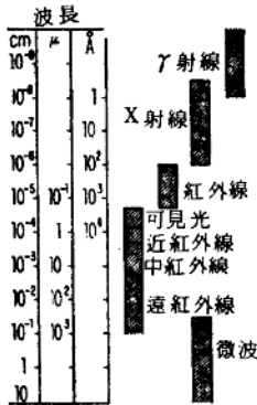
圖 1-2 電磁波譜
