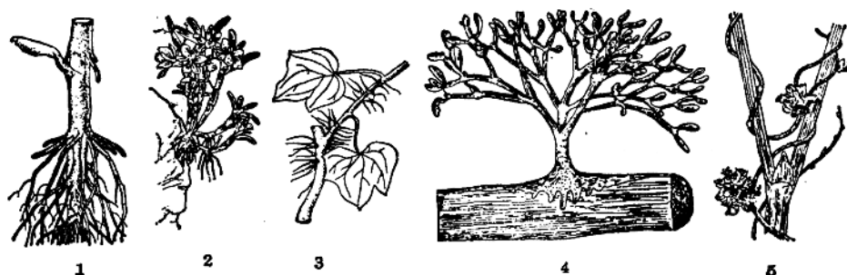
图 1-3 根的变态
