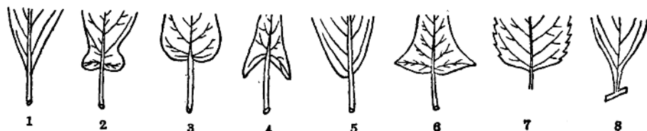
图 1-11 叶基的形状
