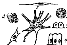
图1-2 细胞的形态
