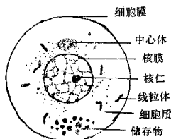
图1-1 细胞
