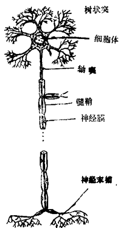
图1-6 神经元
