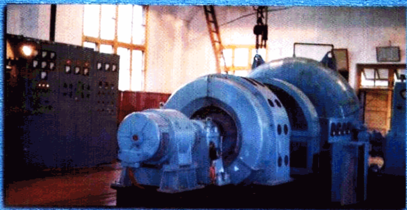
▲官庄水电站发电机组之一 谢磊摄
