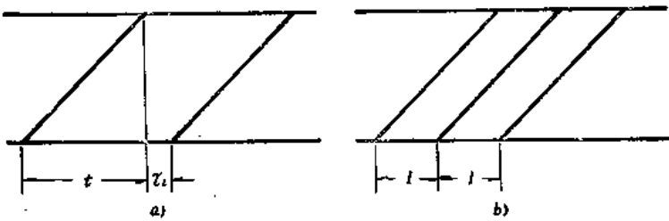
图 2—4 双线平行运行图时间
