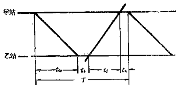
图 2—3 单线平行成对运行图周期
