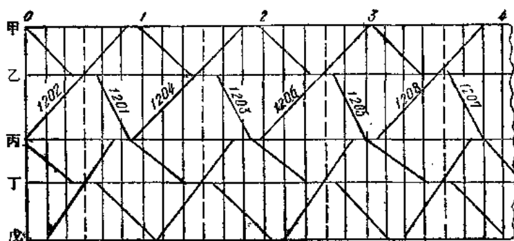
图 2—1 单线平行成对运行图
