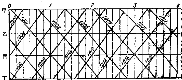
图 2—2 双线平行运行图
