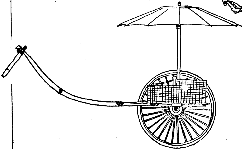
甘肃平凉庙底战国墓出土一号车复原图
