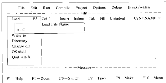
图 5 装入文件屏幕示意图
