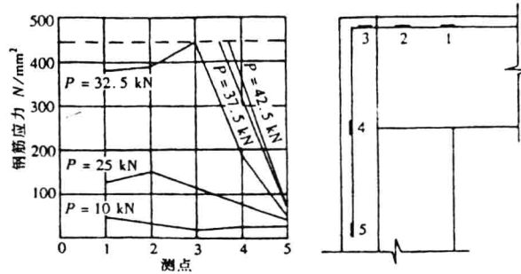
图 6 梁纵筋应力
