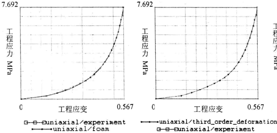
图 1 基于广义 Ogden 模式的拟合曲线与试验曲线比较
