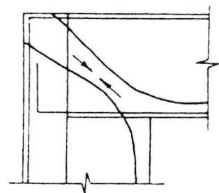
图 7 斜压杆传力原理
