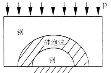
图 4 层合结构
