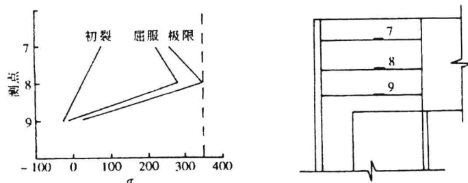
图4 箍筋应力 (N/mm 2 )
