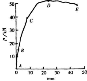
图 5 P-Δ 曲线
