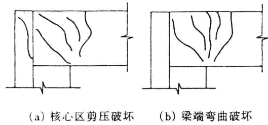
图3 破坏形式
