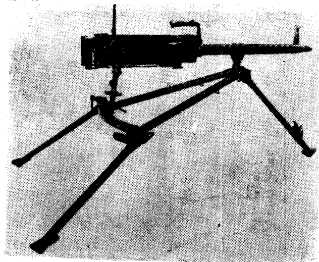
第二十一工厂造气冷式马克沁重机枪
