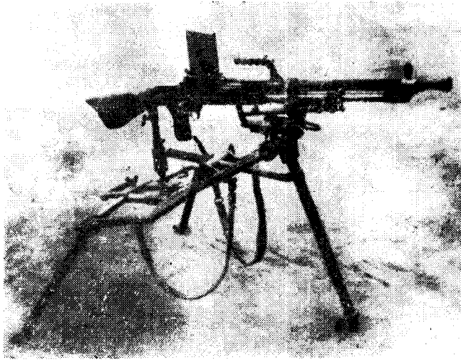
西北制造厂造捷克式轻机枪
