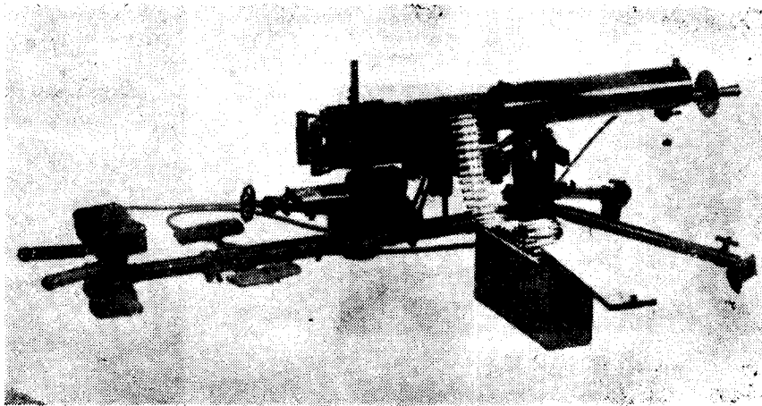
金陵兵工厂造水冷式马克沁重机枪
