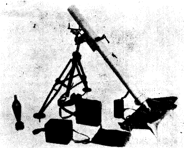
第二十一工厂造82迫击炮
